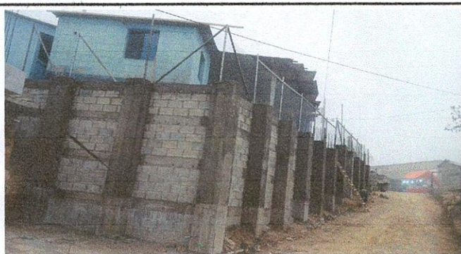
Foto 5: Finalización de muro de contención con reforzamiento de drenes.
