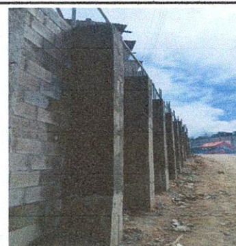
Foto 6: Finalización del mejoramiento de 12 mtr lineales de muro de contención, con zapatas aisladas de 1.20 x 1.20 m, cemento corrido, columnas de concreto y solera de humedad.
